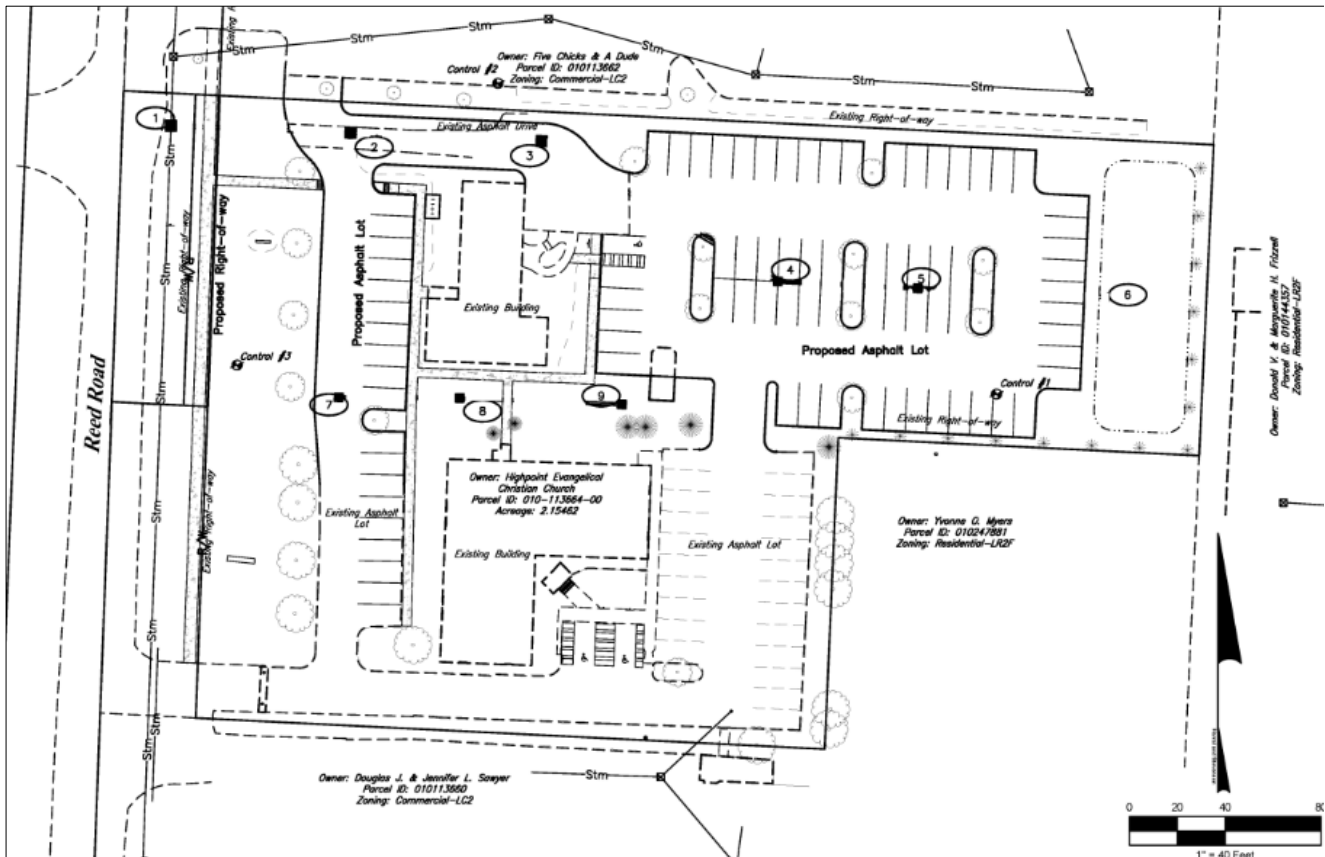
圖 42, 5054 Reed Road 和 5038 Reed Road 的整體配置規劃
