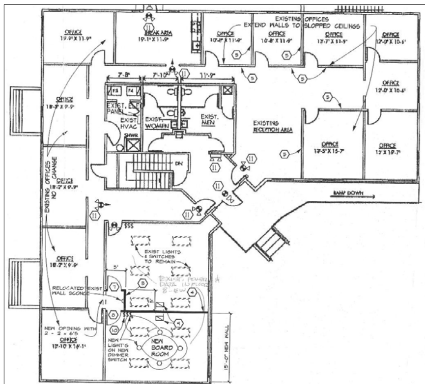
圖 37: 5038 Reed Road 現在 (原有) 上層內部空間配置
