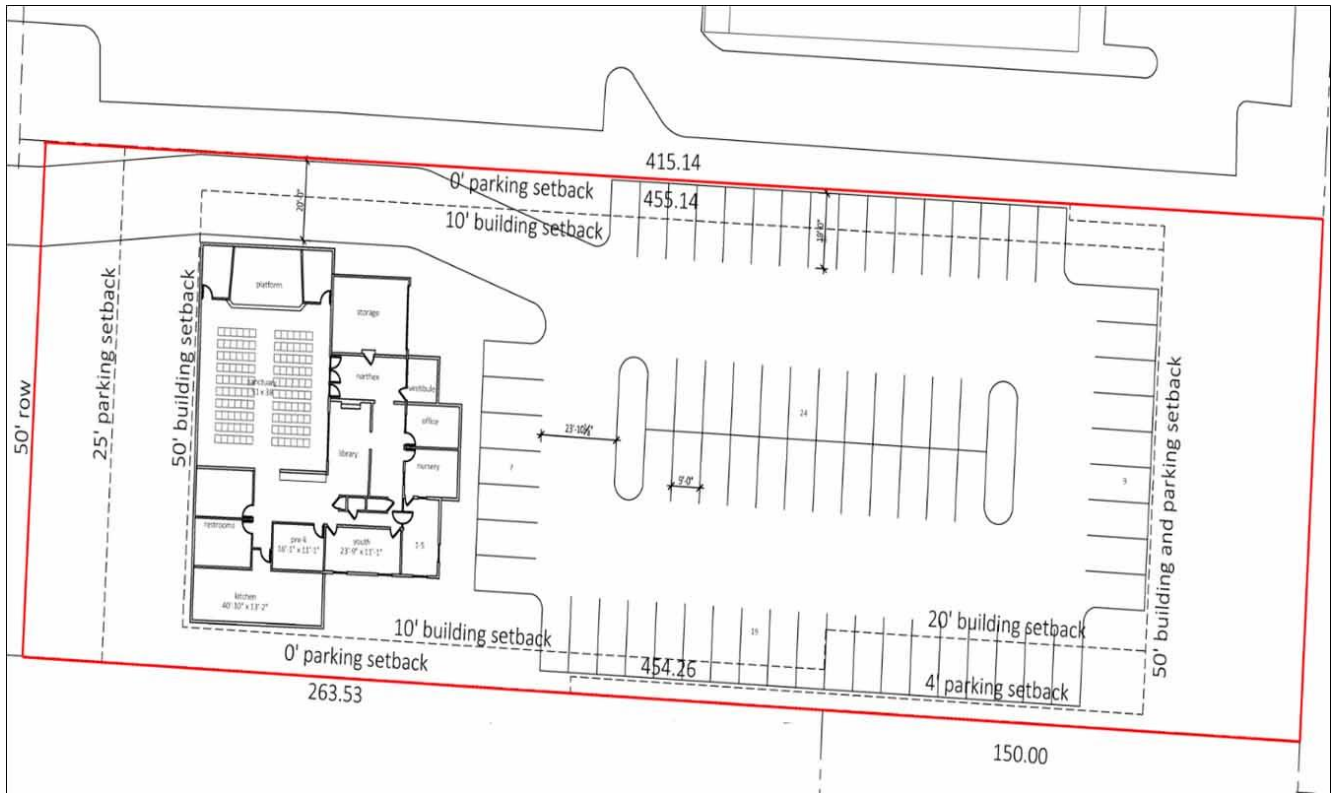
圖 34, 5054 Reed Road 的 Plan A 落實整體的基地計劃
