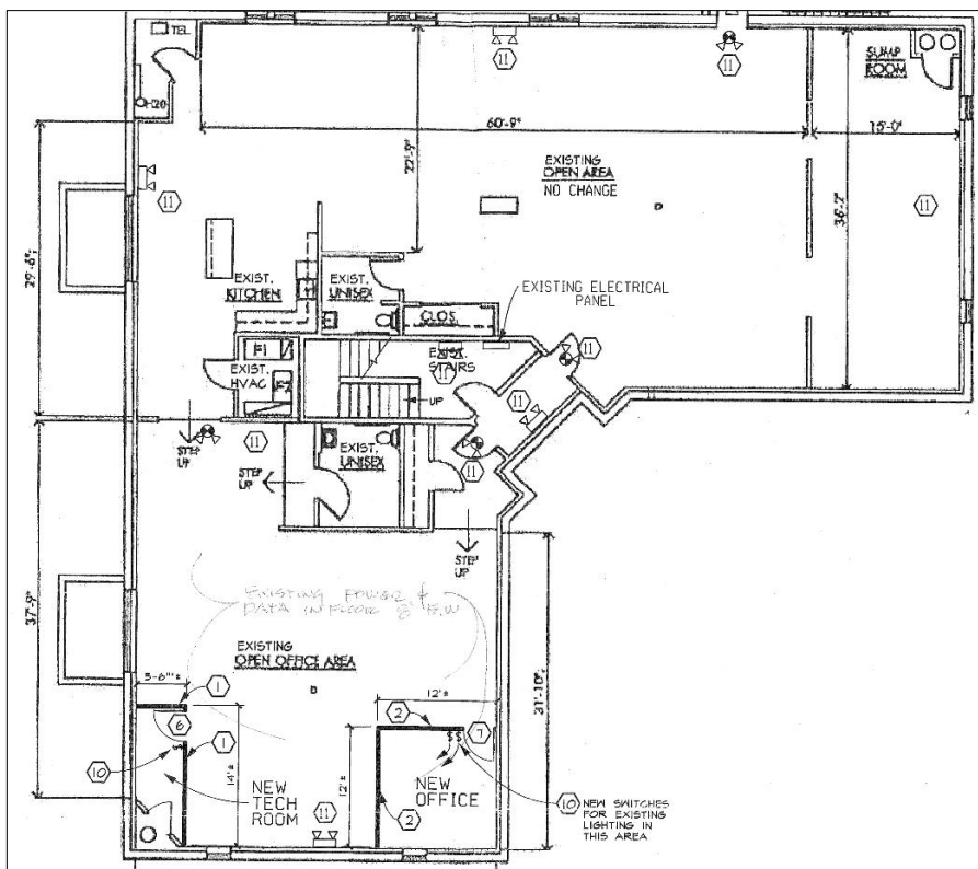
圖 38: 5038 Reed Road 現在 (原有) 底層內部空間配置
