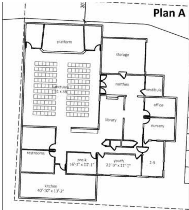
圖 32: 5054 Reed Road 的 Plan A 一樓空間配置
